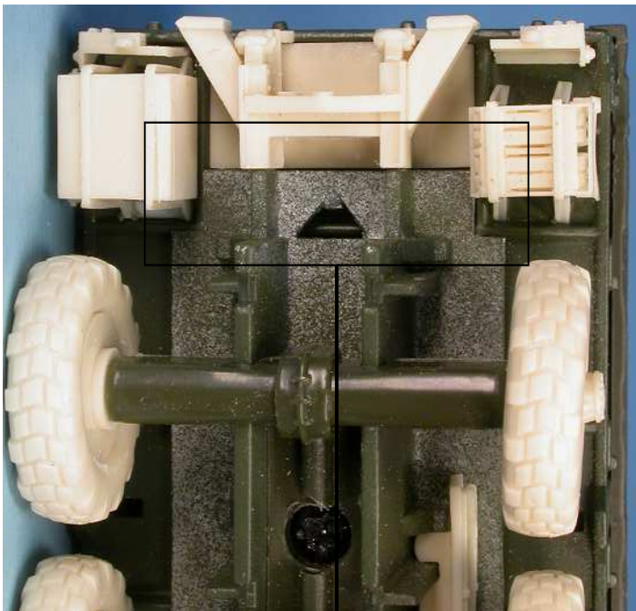
Découpe châssis Solido Cut the Solido chassis
