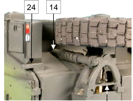
Tige laiton rod brass ø 2 mm
