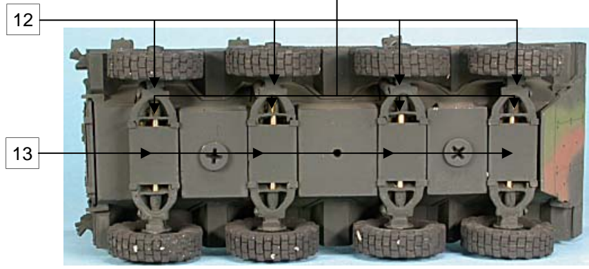
Tige laiton rod brass ø 2 mm
