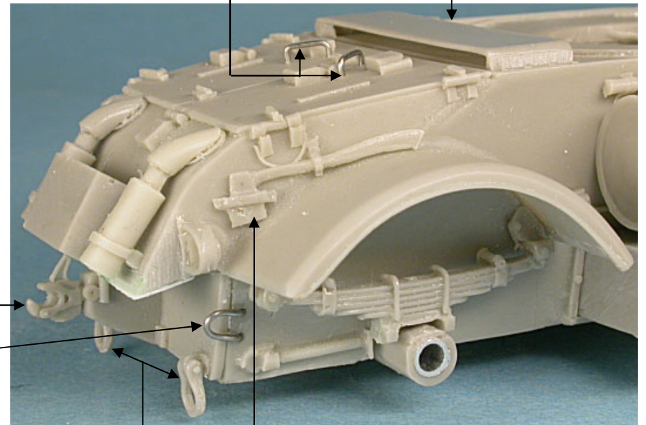
Tige laiton / Brass rod ø 0.5 mm
