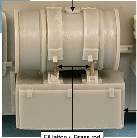
Fil laiton / Brass rod ø 0.5 mm
