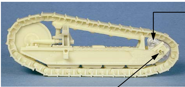
Tige laiton / rod brass \varnothing 1.2 mm
