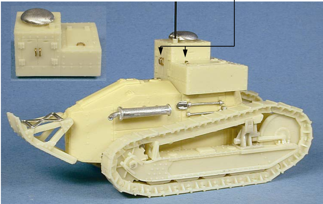
Tige laiton / rod brass \varnothing 0.5 mm
