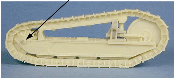
Tige laiton / rod brass \varnothing 1.2 mm
