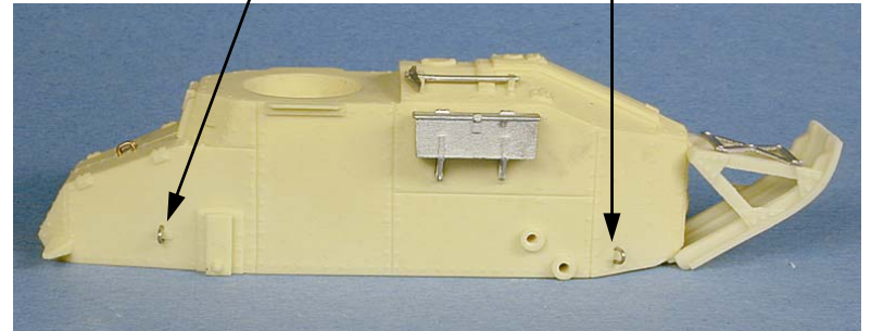
Tige laiton / rod brass ø 0.5 mm
